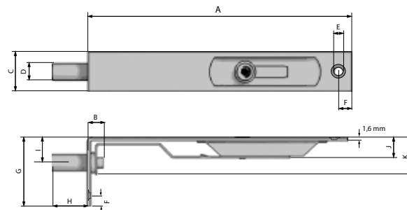
Cuadro de medidas (mm)
