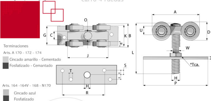
Cuadro de medidas (mm)
